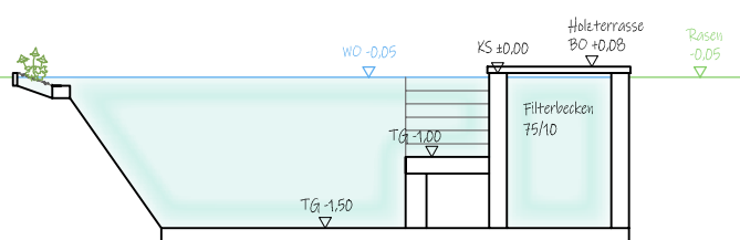
Schema: Schnitt Naturpool mit Pflanzbereich (gemauert & gegraben)
