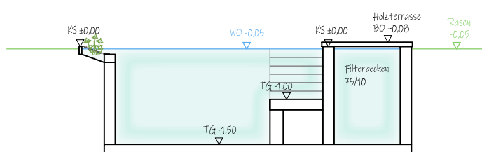
Schema: Schnitt Naturpool mit Pflanzbereich
