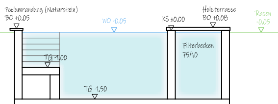
Schema: Schnitt Naturpool mit Stiege
