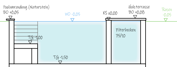
Schema: Schnitt Naturpool mit Stiege
