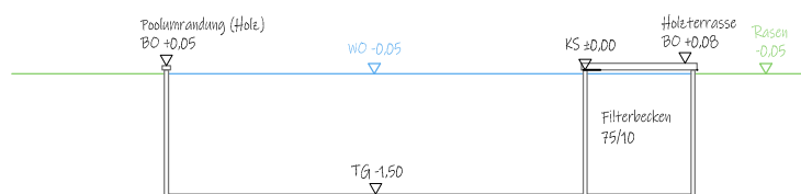
Schema: Schnitt Teco-Fertig-Naturpool
