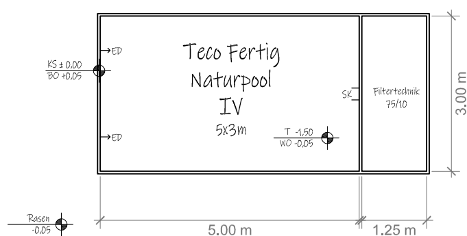
Teco-Fertig-Naturpool ohne Poolumrandung
