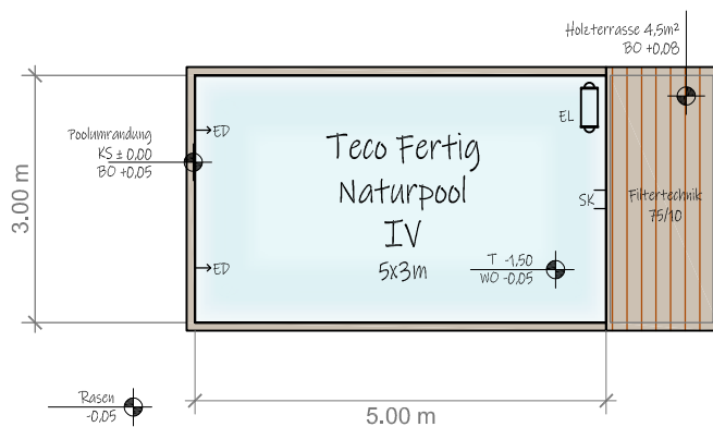
Teco-Fertig-Naturpool mit Poolumrandung (Holz)
